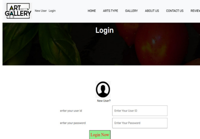
Fig.1 admin module
