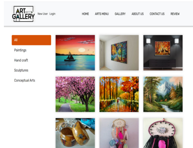
Fig.2user module
